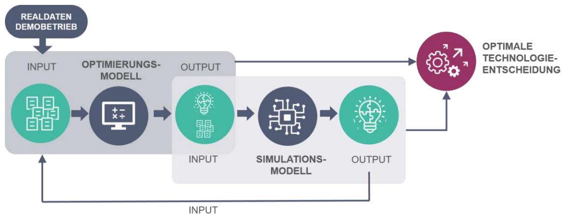
Abbildung 3 Technologieentscheidungs-Prozess
